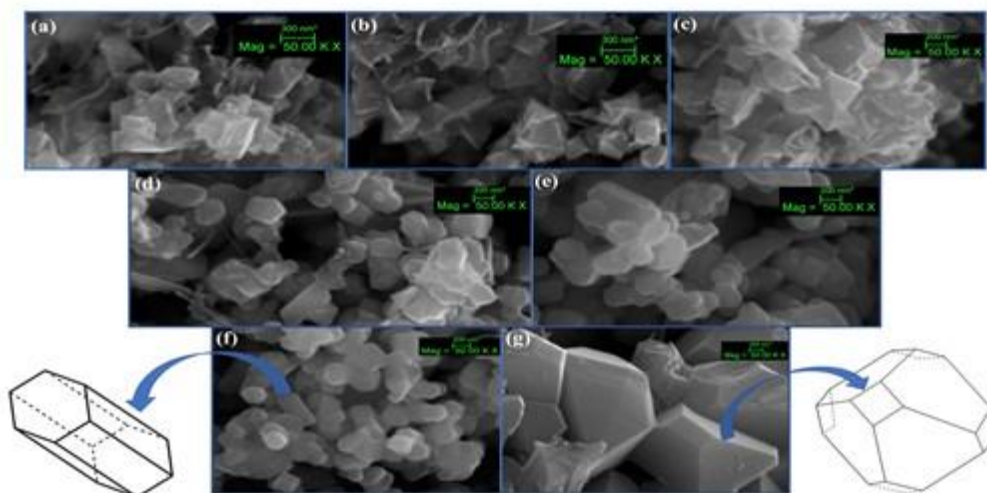
Figure 8: SEM of (a) MnO, (b) MnO 160 °C, (c) MnO 480 °C, (d) MnO 715 °C, (e) MnO 870 °C, (f) MnO 920 °C and (g) MnO 1150 °C samples.
